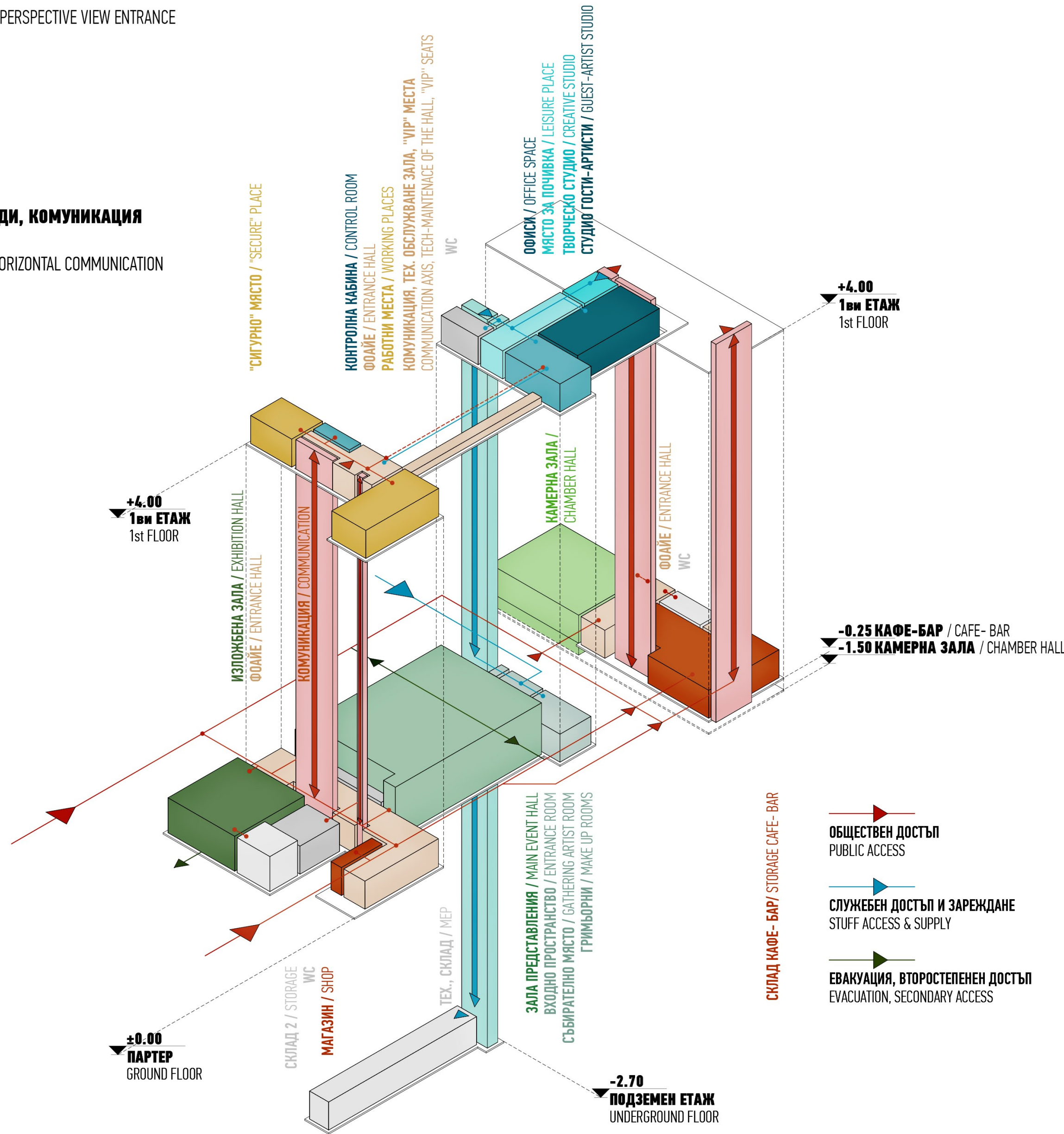
ПЕРСПЕКТИВЕН ИЗГЛЕД ГЛАВЕН ВХОД / PERSPECTIVE VIEW ENTRANCE
